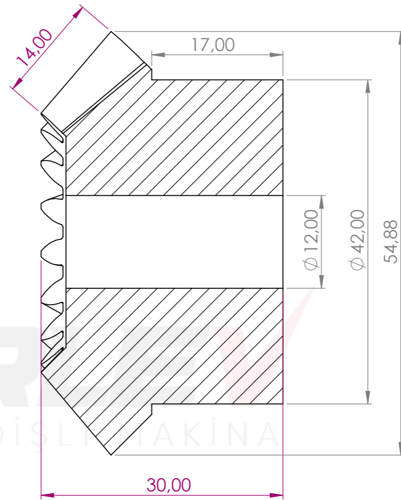
KESİT A-A ÖLÇEK 2 : 1
