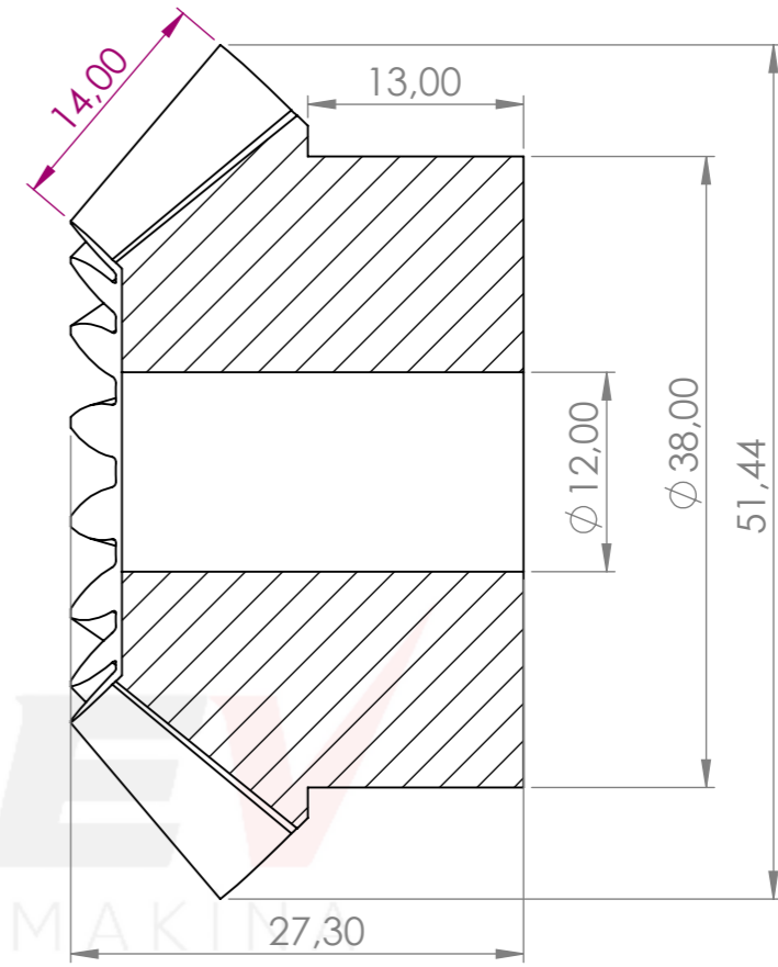
KESİT A-A
