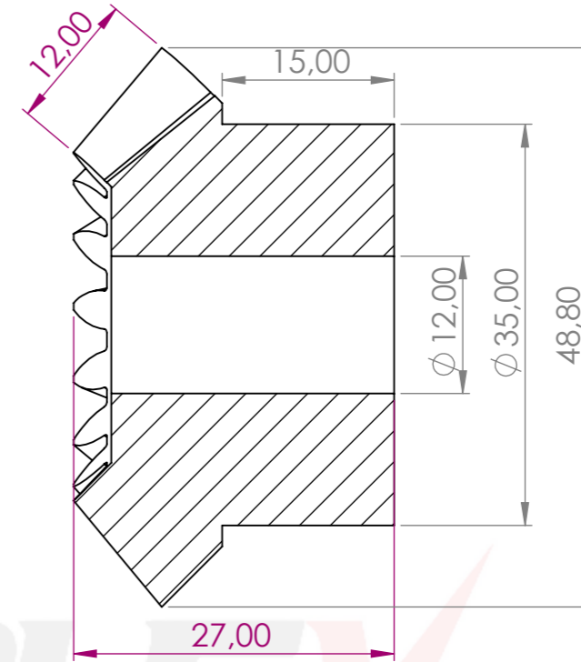
KESIT B-B ÖLÇEK 2 : 1.2
