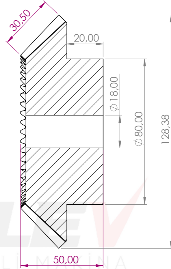
KESİT A-A ÖLÇEK 1 : 1.2
