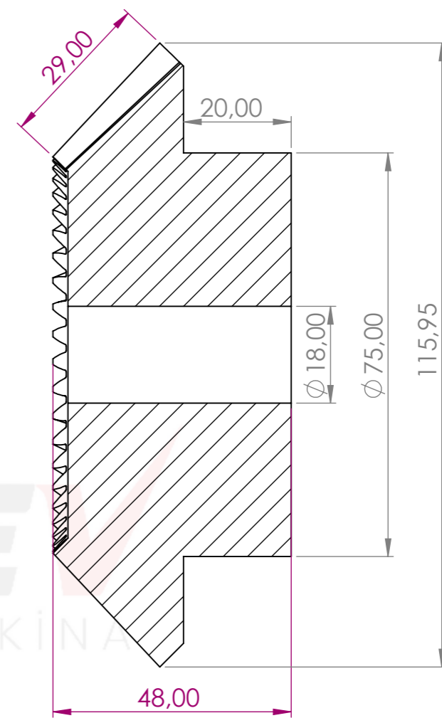
KESİT A-A
