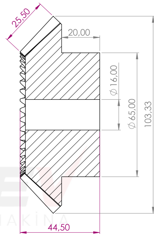
KESİT A-A
