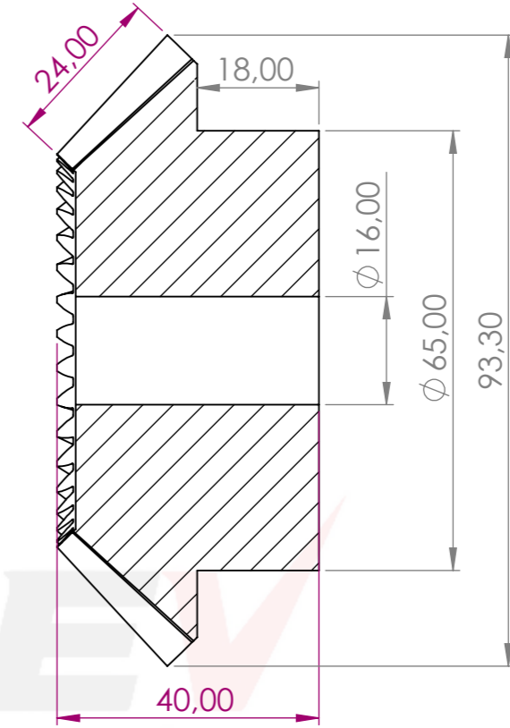
KESİT A-A
