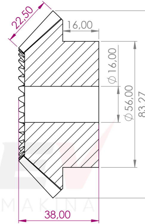
KESİT A-A
