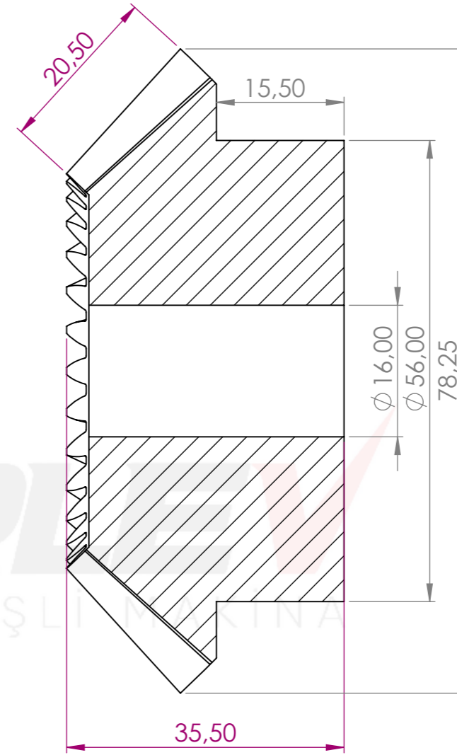
KESİT A-A ÖLÇEK 2 : 1.3
