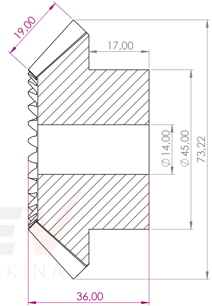
KESİT A-A ÖLÇEK 2 : 1.3
