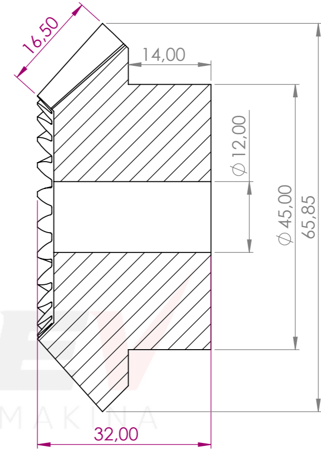
KESİT A-A ÖLÇEK 2 : 1.3
