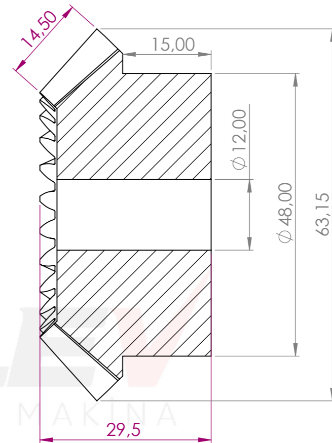
KESİT A-A ÖLÇEK 2 : 1.3
