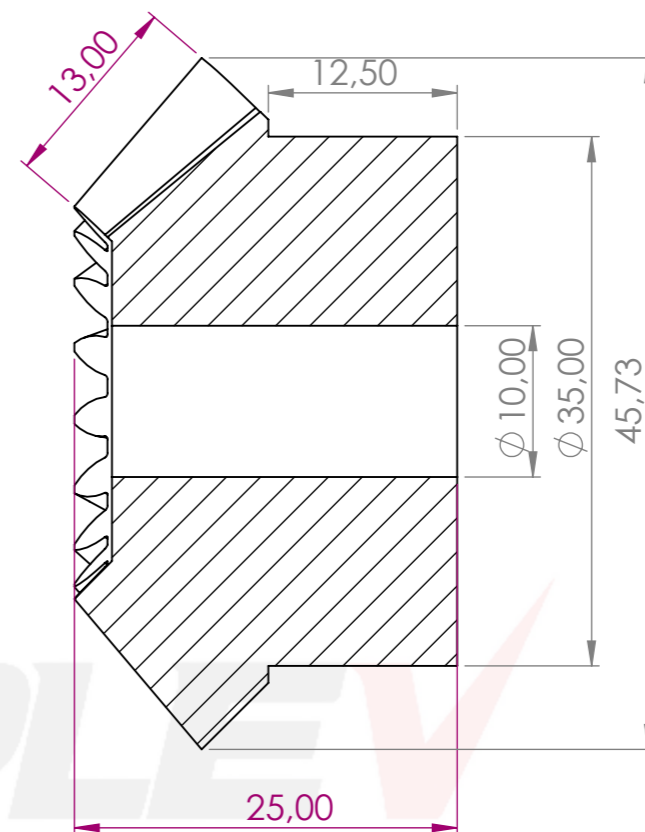
KESİT A-A
