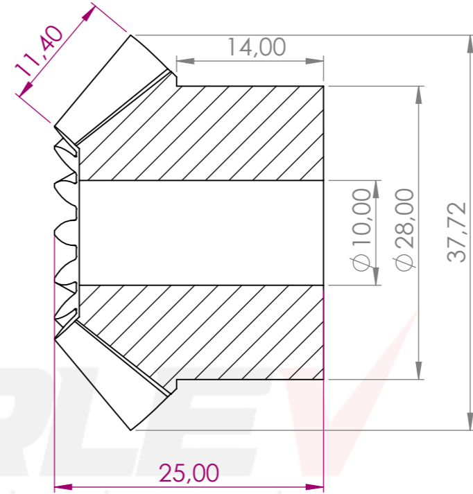
KESİT A-A
