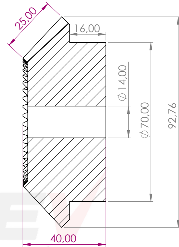
KESİT A-A
