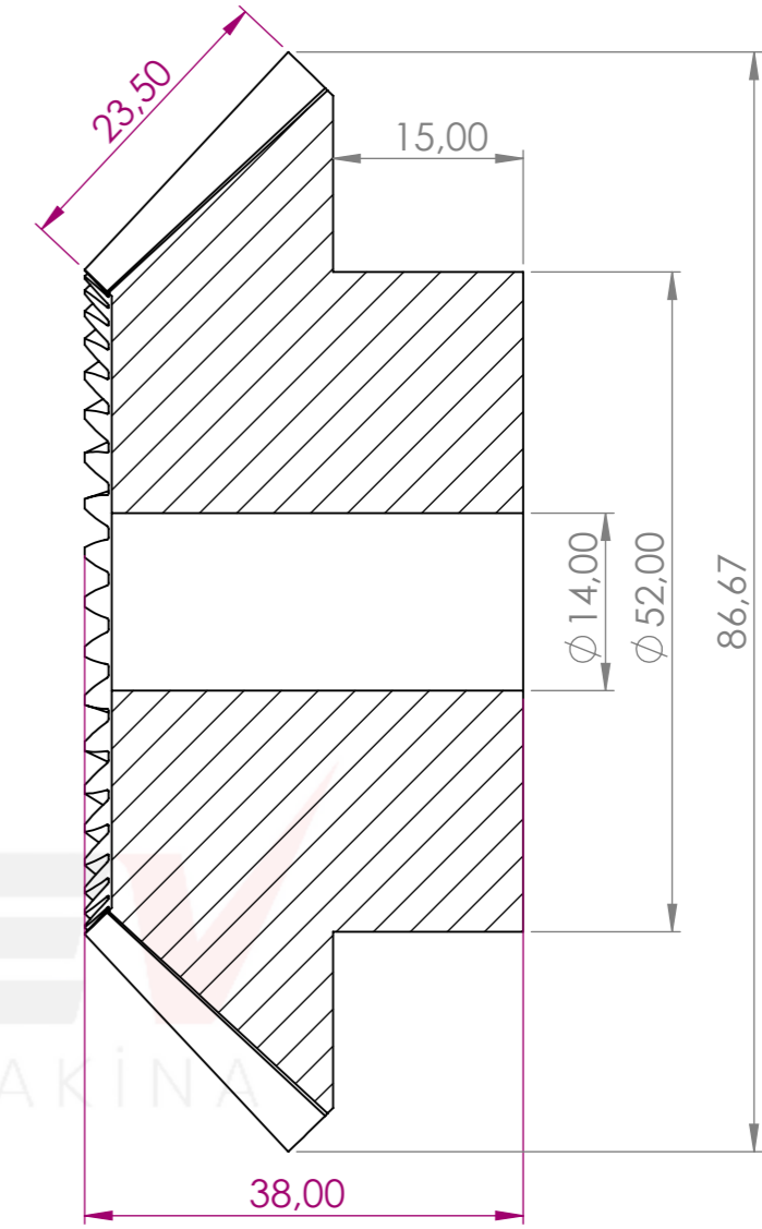
KESİT A-A ÖLÇEK 2 : 1.3
