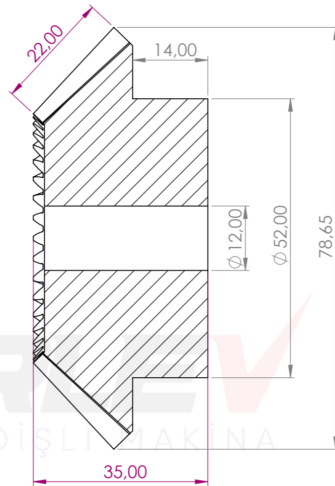
KESİT A-A ÖLÇEK 2 : 1.4
