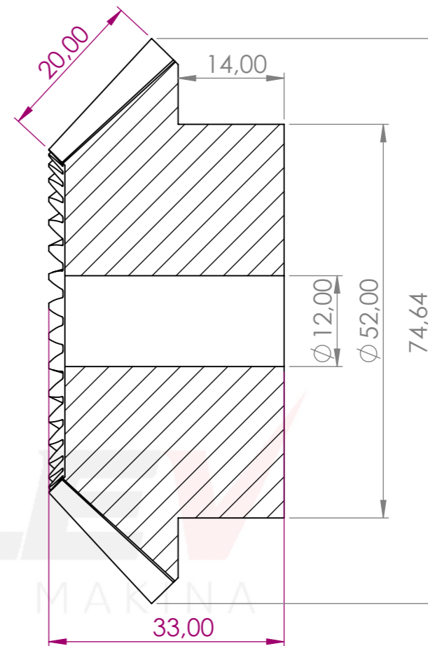
KESİT A-A ÖLÇEK 2 : 1.4
