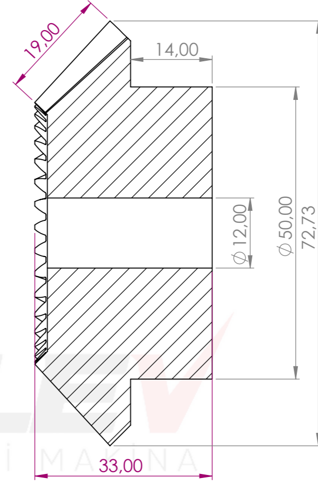
KESİT A-A ÖLÇEK 2 : 1.3
