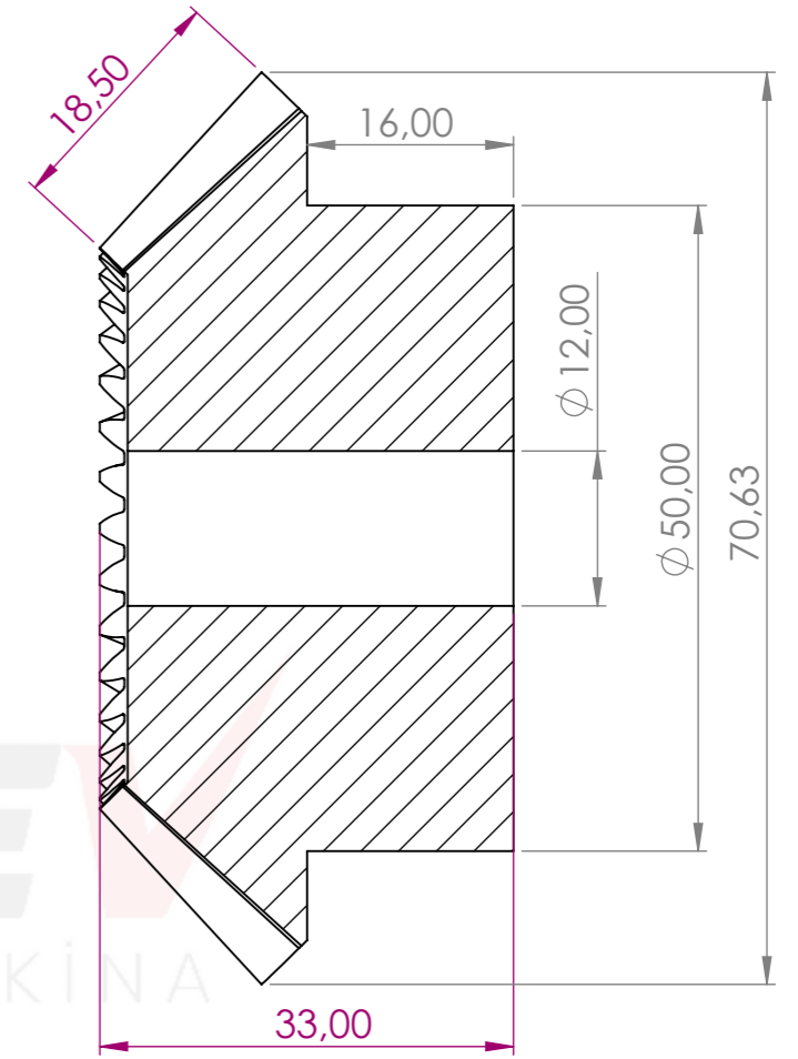
KESİT A-A ÖLÇEK 2 : 1.3
