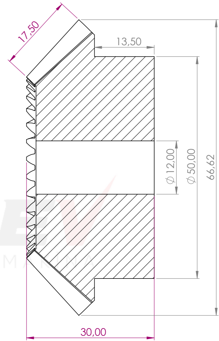
KESİT A-A ÖLÇEK 2 : 1
