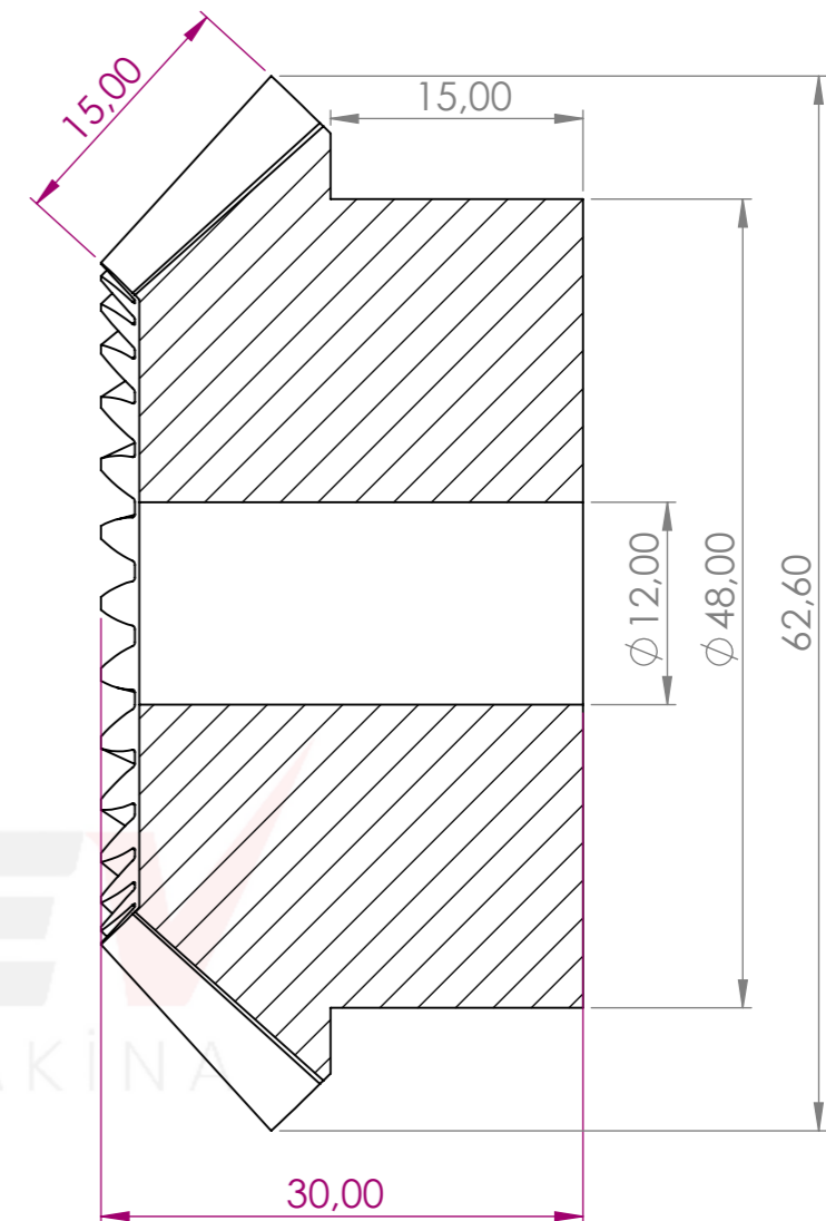
KESİT A-A ÖLÇEK 2 : 1
