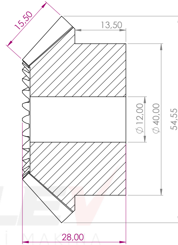
KESİT A-A ÖLÇEK 2:1
