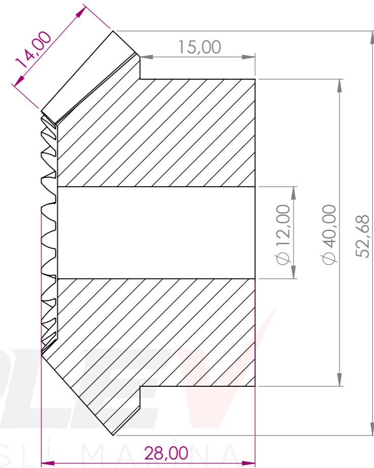
KESİT A-A
