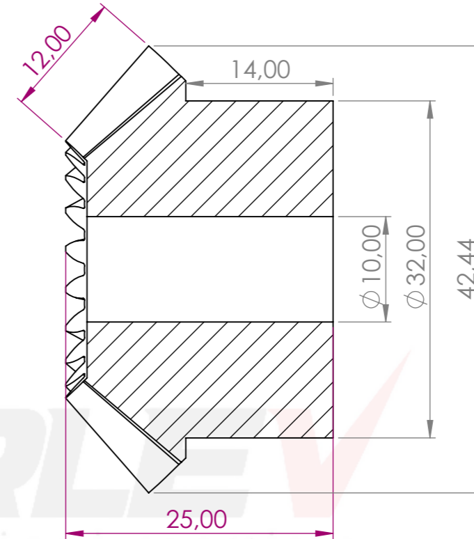
KESİT B-B
