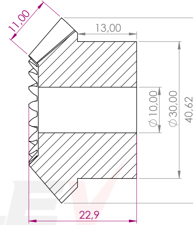
KESİT A-A
