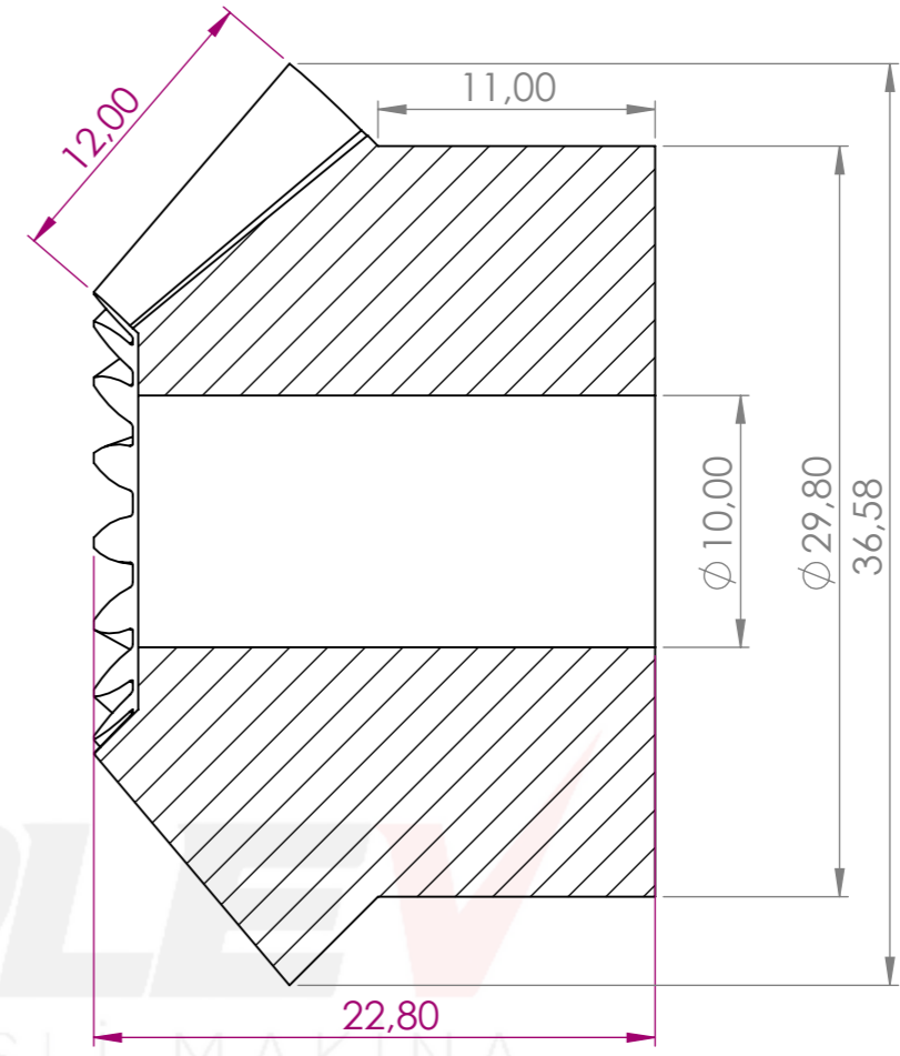
KESİT A-A ÖLÇEK 3 : 1
