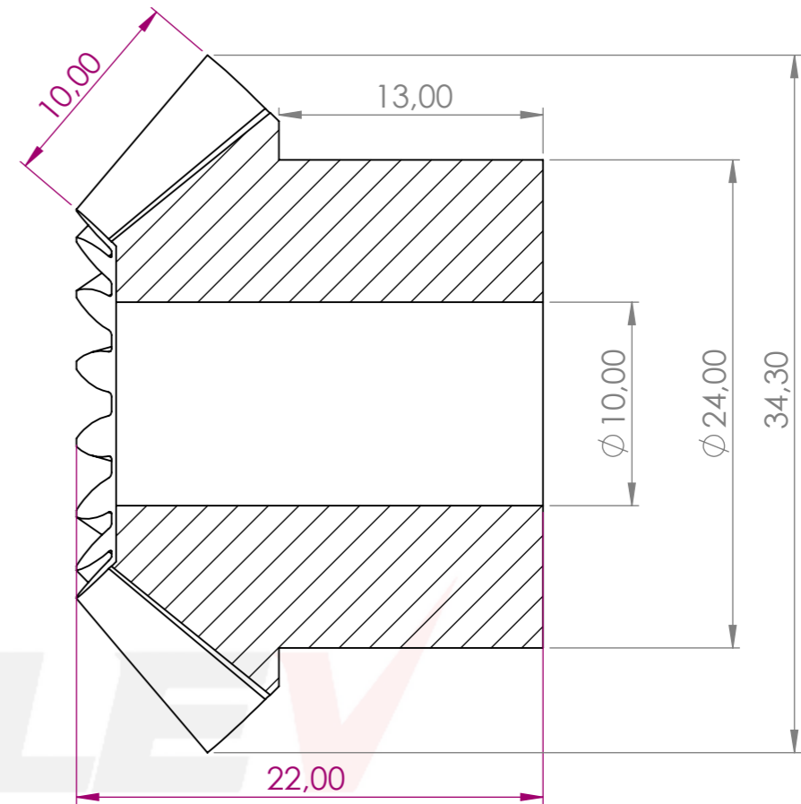
KESİT A-A ÖLÇEK 3 : 1
