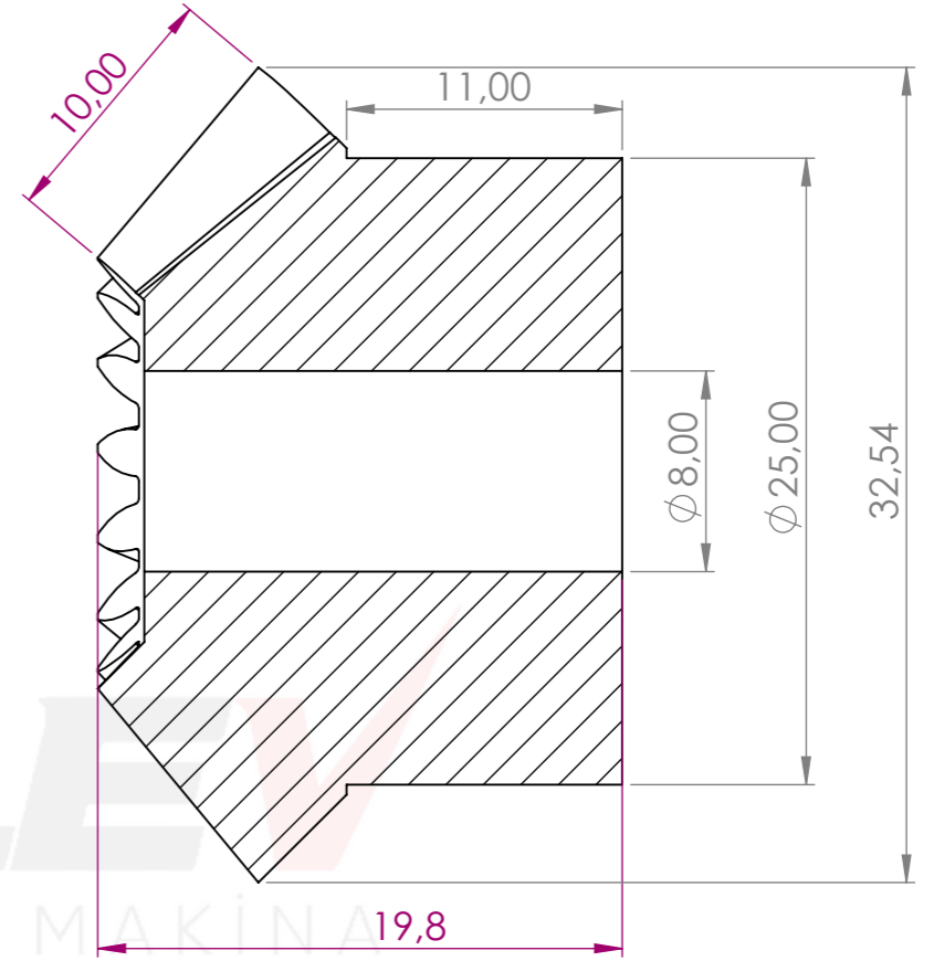
KESİT A-A ÖLÇEK 3 : 1
