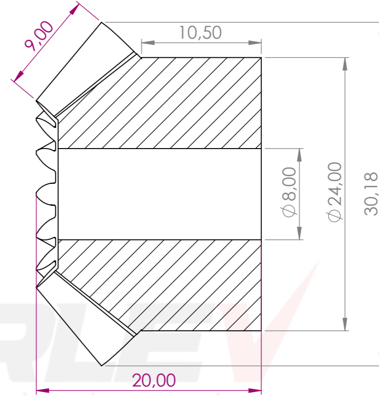
KESİT A-A ÖLÇEK 3 : 1
