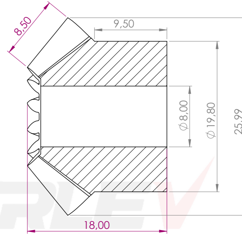
KESİT A-A ÖLÇEK 5 : 1.5
