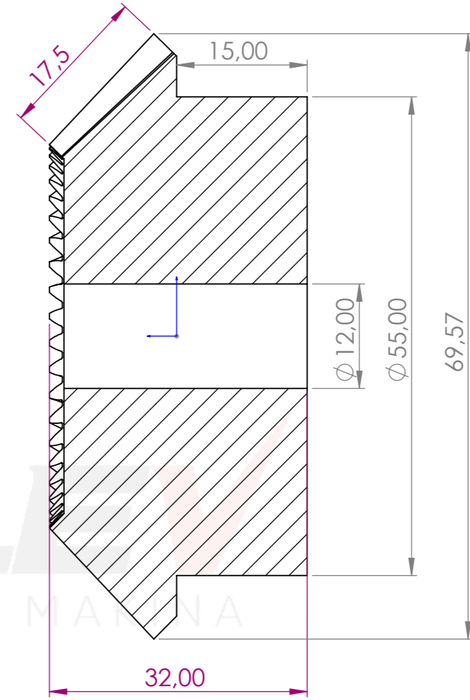
KESİT A-A ÖLÇEK 2 : 1.2
