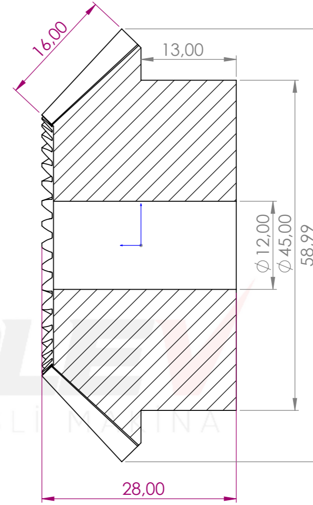
KESİT A-A ÖLÇEK 2 : 1
