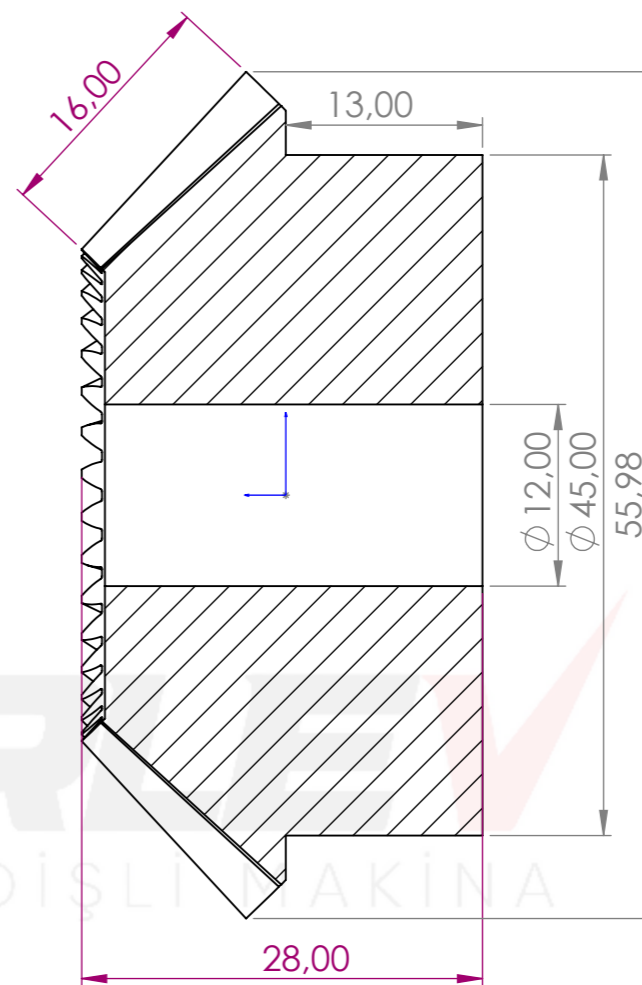
KESİT A-A ÖLÇEK 2 : 1
