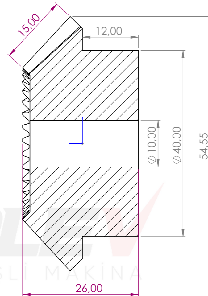
KESİT A-A
