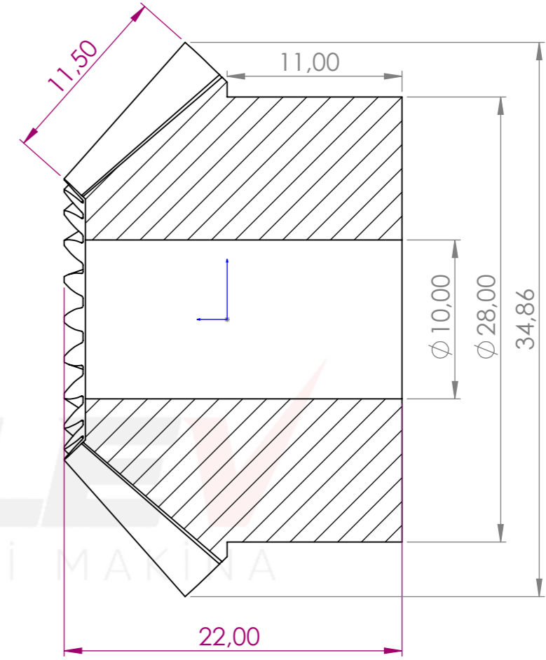
KESIT A-A ÖLÇEK 3 : 1
