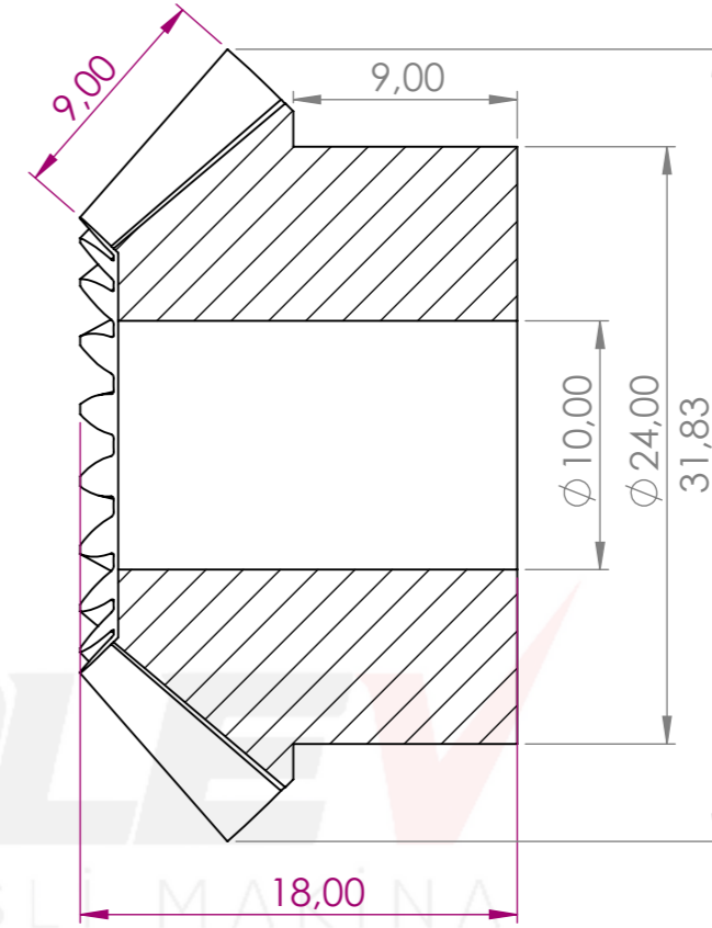
KESİT A-A ÖLÇEK 3 : 1
