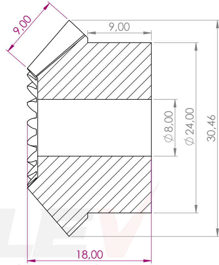
KESİT A-A ÖLÇEK 3:1
