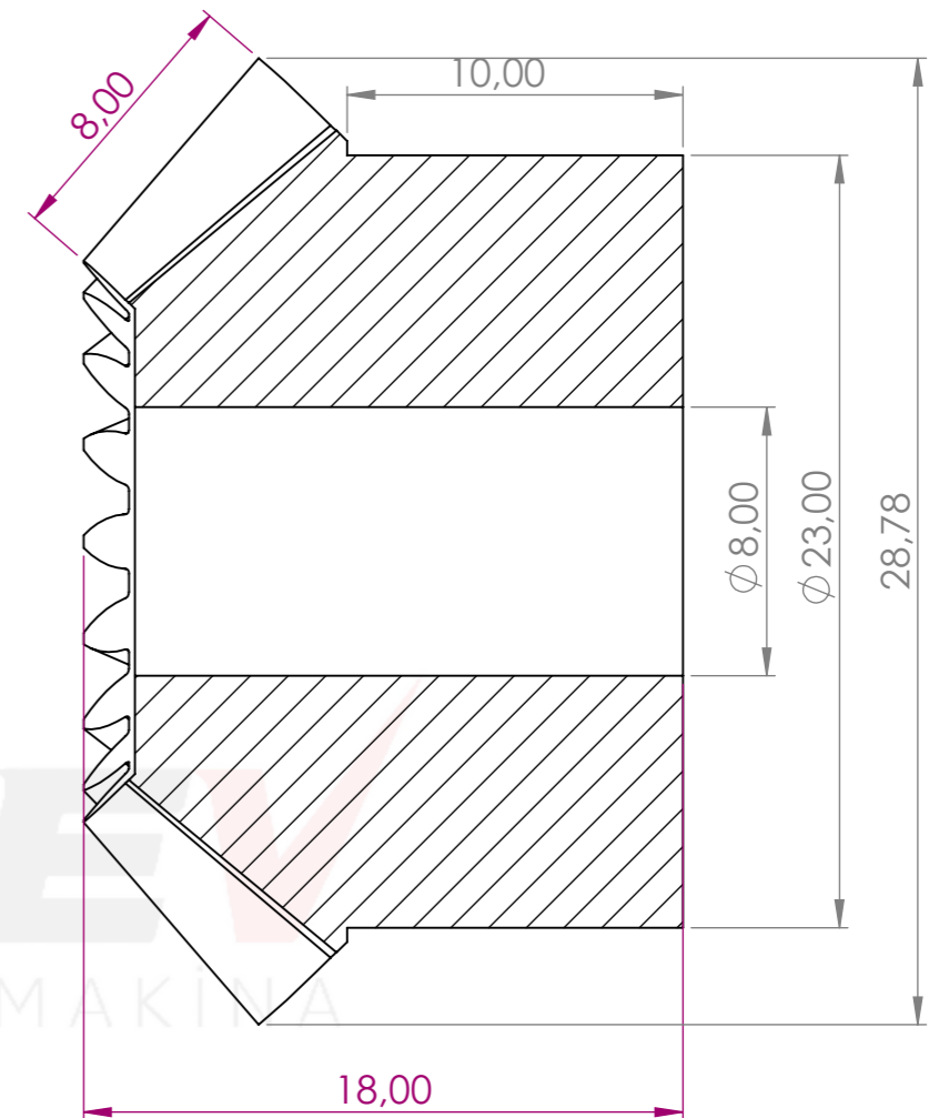
KESİT A-A ÖLÇEK 4 : 1
