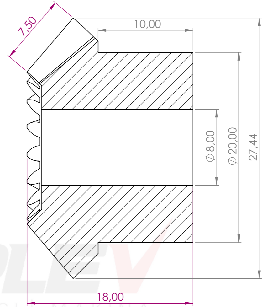
KESİT A-A ÖLÇEK 4 : 1
