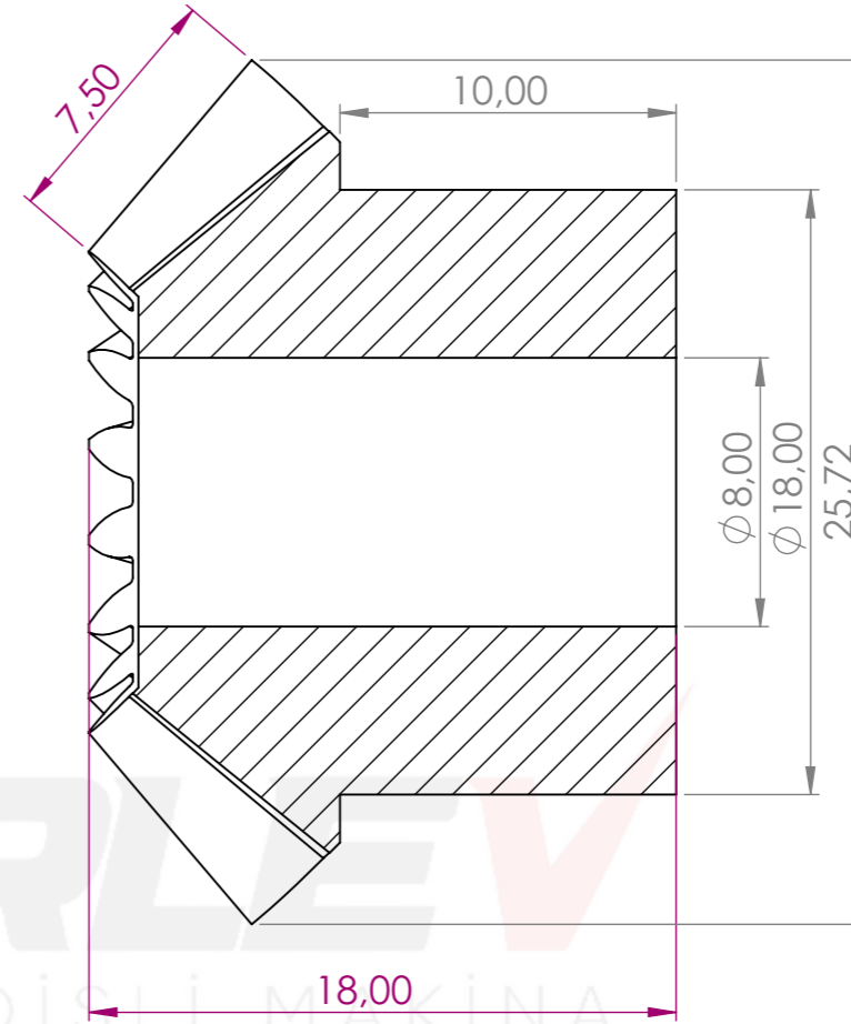
KESİT A-A ÖLÇEK 4 : 1
