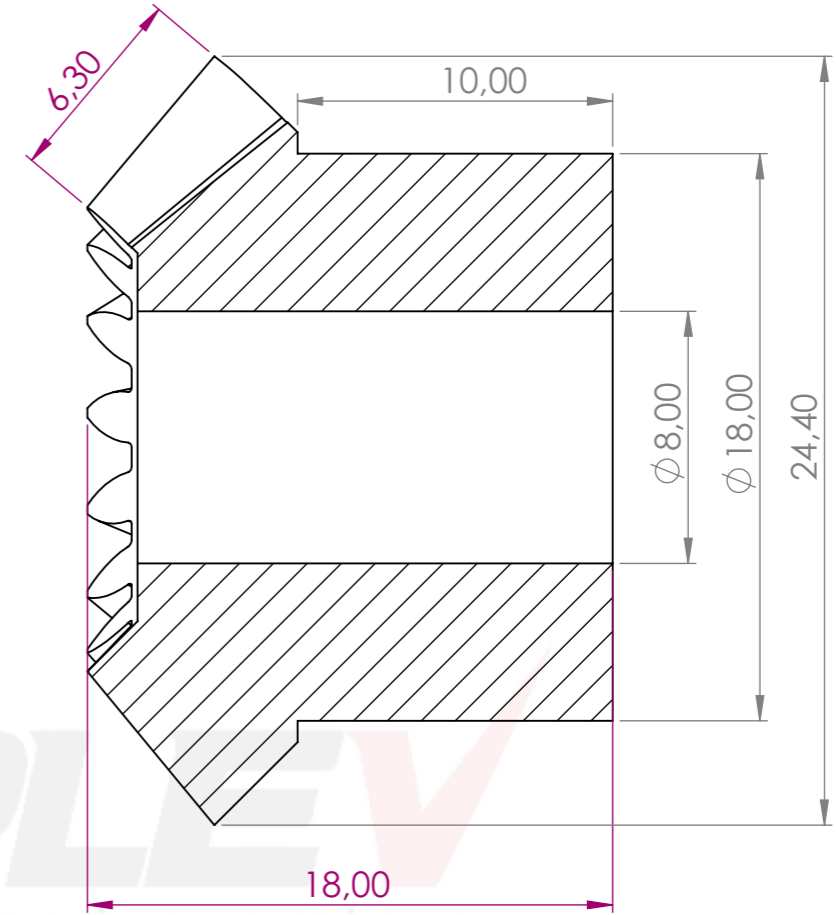
KESİT A-A ÖLÇEK 5 : 1.2
