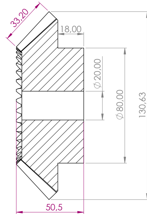
KESİT A-A ÖLÇEK 1 : 1.3
