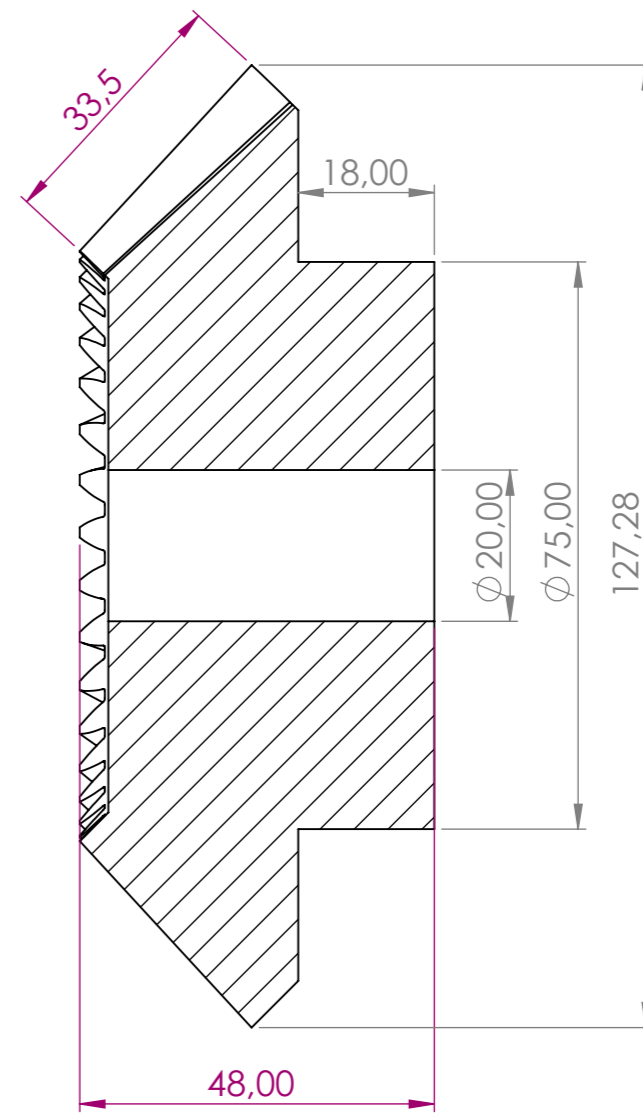
KESİT A-A ÖLÇEK 1:1
