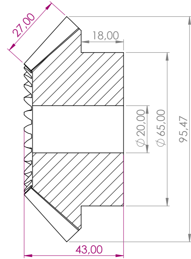
KESİT A-A
