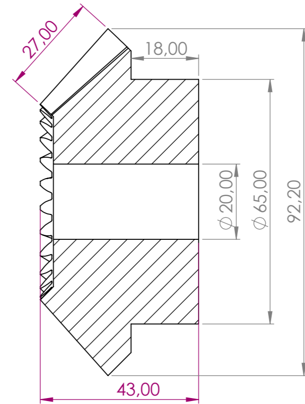
KESİT A-A
