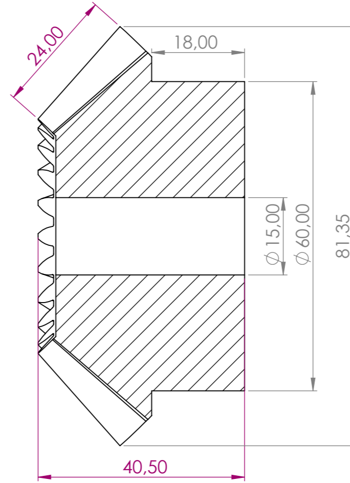
KESİT A-A ÖLÇEK 2 : 1.5
