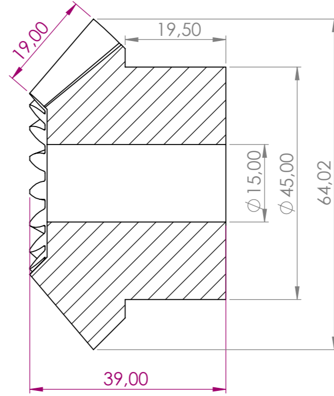
KESİT A-A ÖLÇEK 2 : 1.5
