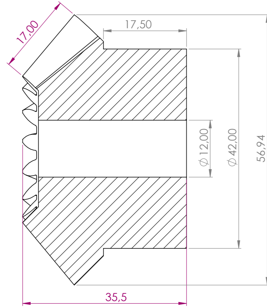
KESİT A-A ÖLÇEK 2 : 1
