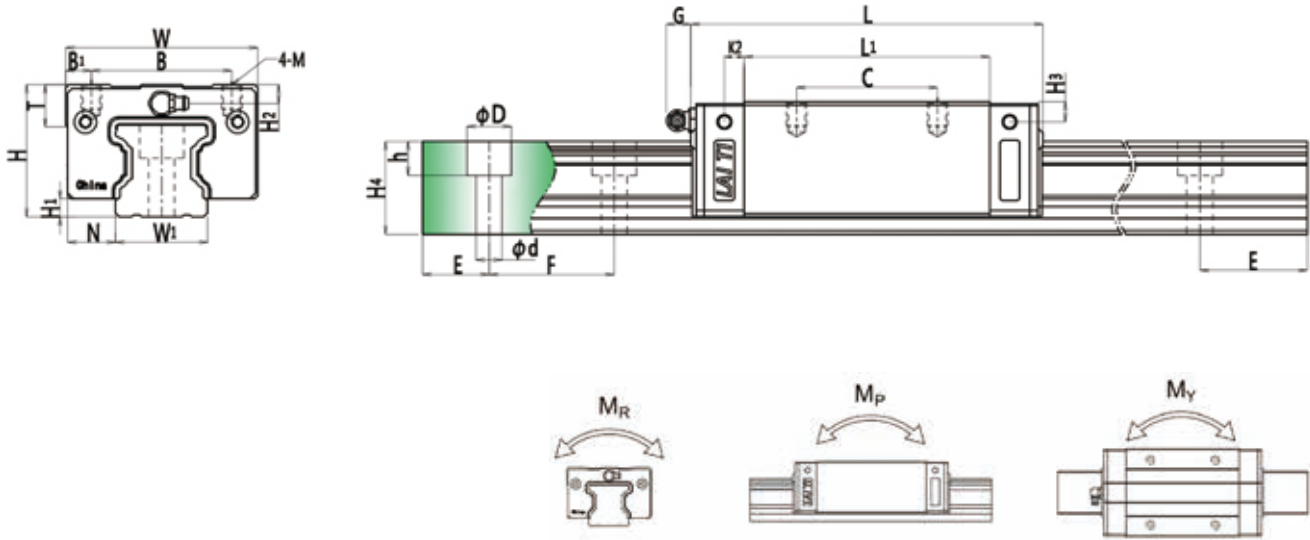
Linear Guide parameter
