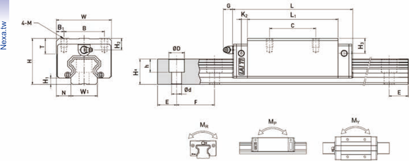
Linear Guide parameter
