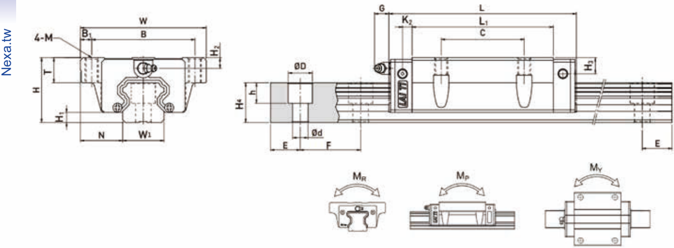
Linear Guide parameter
